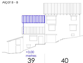
Alçat B - B
